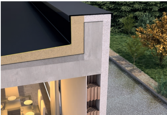
Przekrój dachu płaskiego
